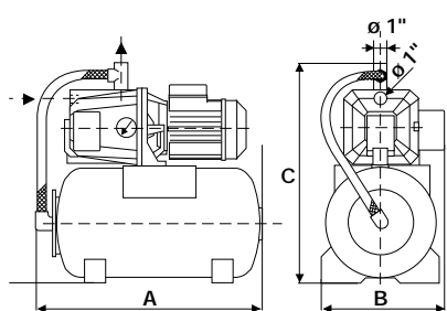
AQUAJET 102/-60-80
