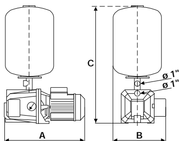
AQUAJET 102/-60-80
